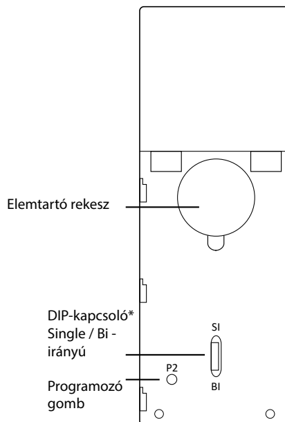
Kézi adó - hátul nyitott fedéllel
