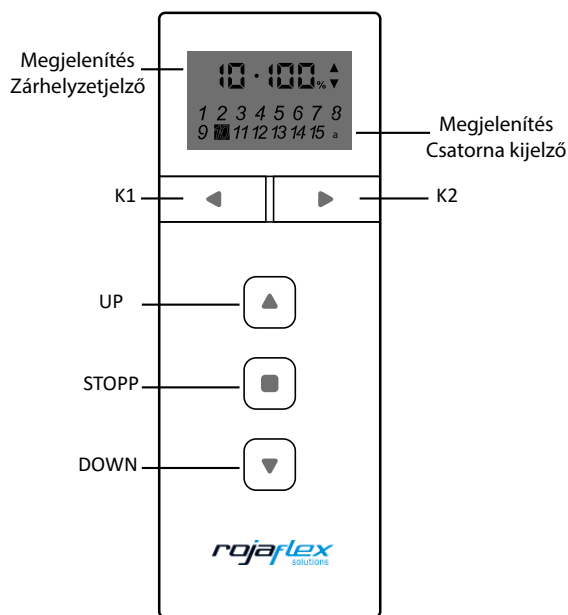
15 csatornás kézi adó HSR-15
