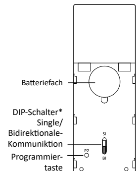
Handsender – Rückseite bei geöffnetem Deckel
