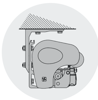
Deckenmontage
