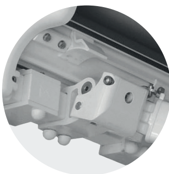
Armhalter
