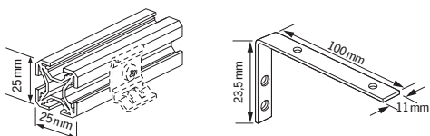
Montageprofil mit Winkel
