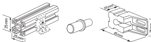
Montageprofil mit Bolzen
