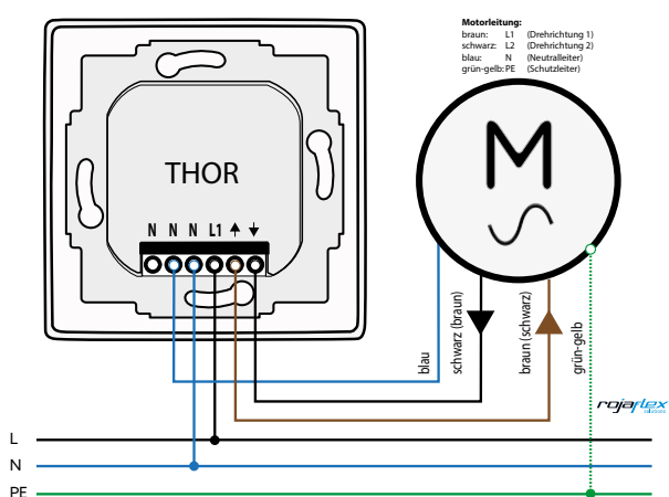
Rohrmotoren mit Rollladen-Zeitschaltuhr Thor
