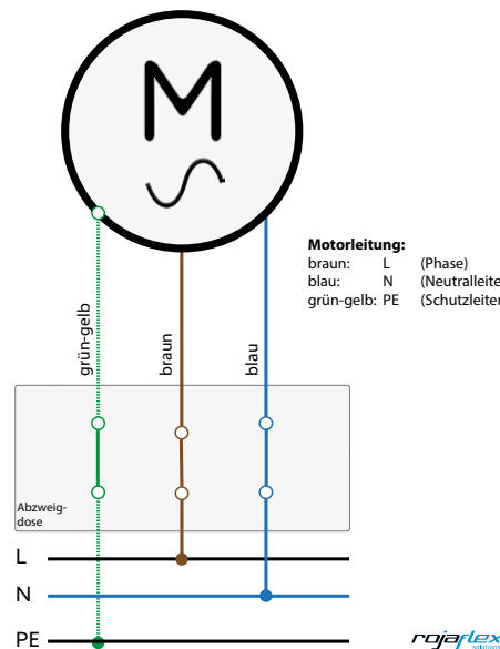
Rohrmotoren mit mechanischen Endschaltern und Funk
