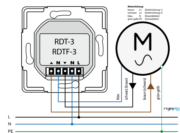
Rohrmotoren mit Rollladen-Zeitschaltuhr RDT-3 / RDTF-3
