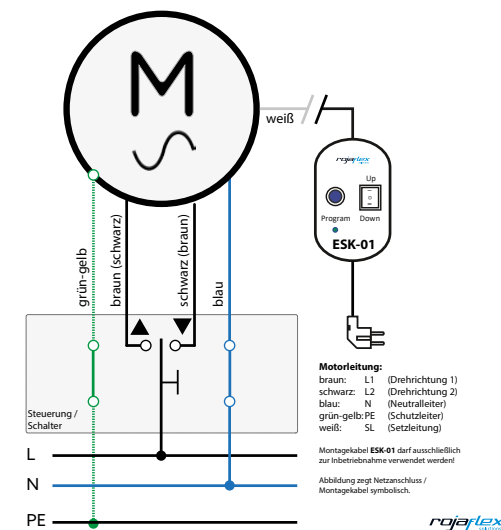
Rohrmotoren mit elektronischen Endschaltern
