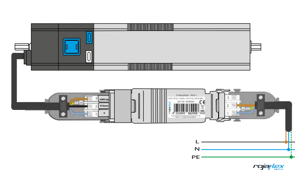
Jalousieantrieb RJM mit Hirschmann-Stecker und Kupplung
