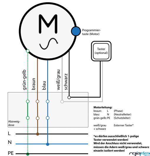
Rohrmotoren mit elektronischen Endschaltern und Funk
