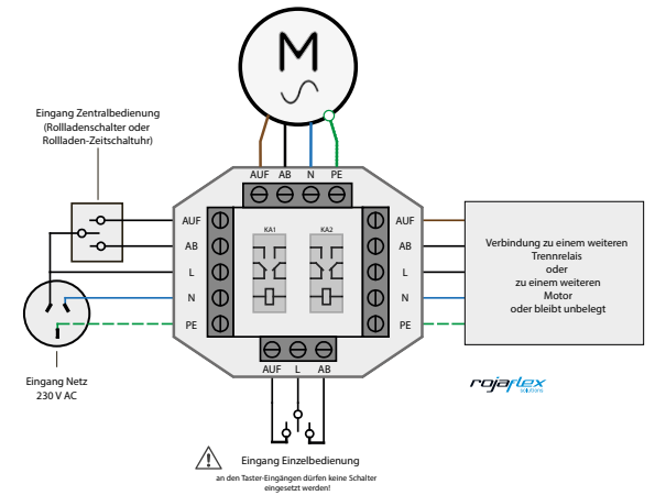
Trennrelais RF-230-R2 für 230 V ~ Antriebe (ohne Funk)
