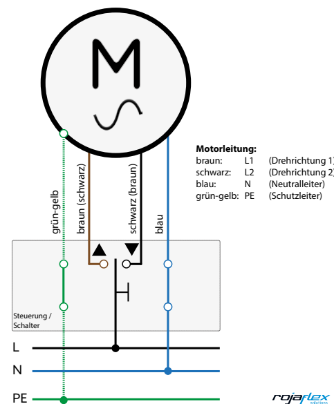
Rohrmotoren mit mechanischen Endschaltern
