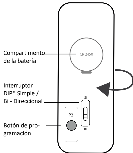
Emisor de mano - parte trasera con la tapa abierta
