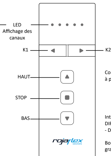
Émetteur à main 5 canaux HSR-5
