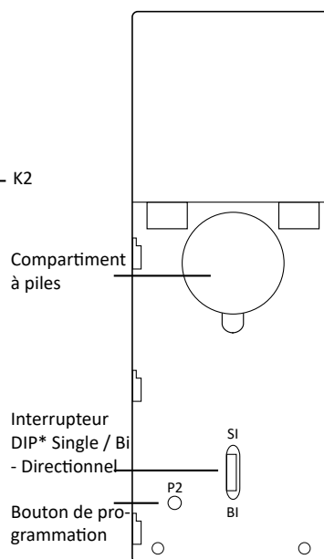
Émetteur portable - face arrière lorsque le couvercle est ouvert
