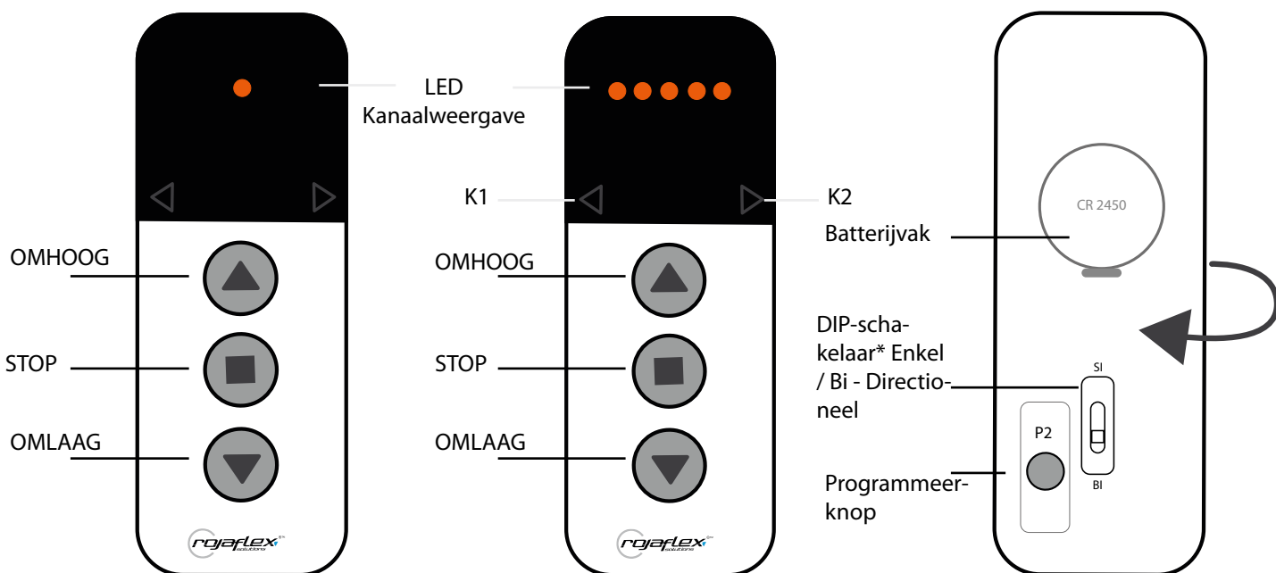
1-kanaals handzender RHS1-W
